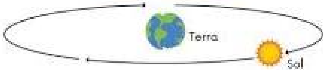
Modelo geocêntrico
