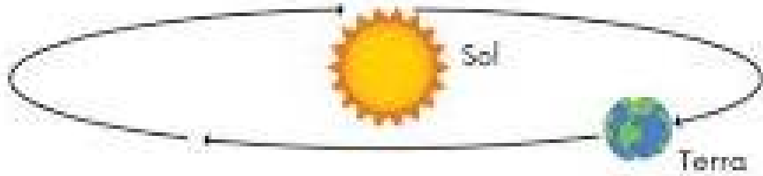
Modelo heliocêntrico
